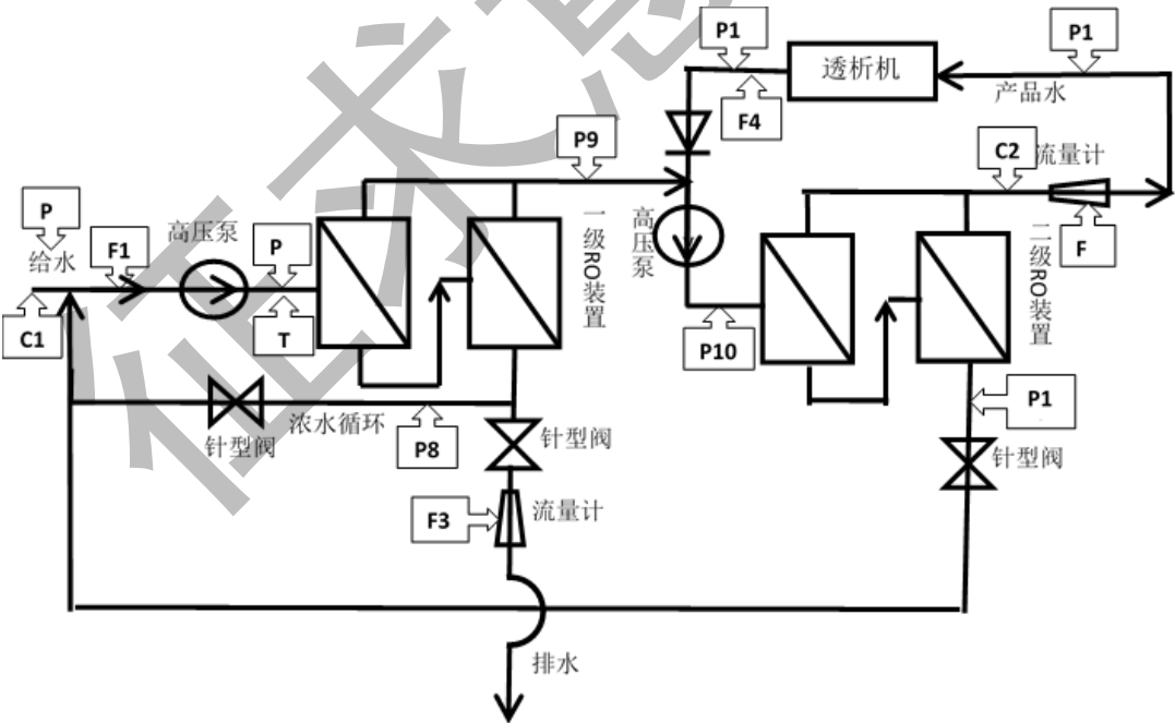
图 1. 反渗透主机检测压力、电导率和水量示意图
