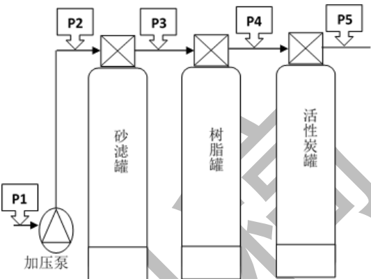
图 1. 预处理部分检测压力示意图
