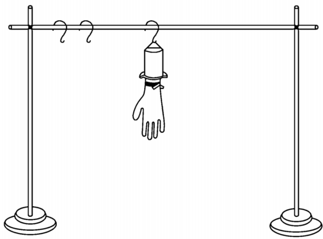
图 A.2 固定装置
